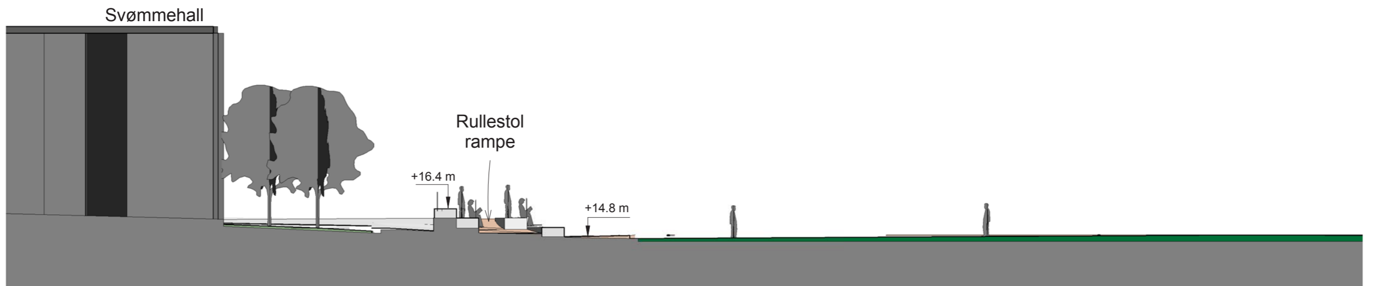
2 Snitt 2 1 : 200
