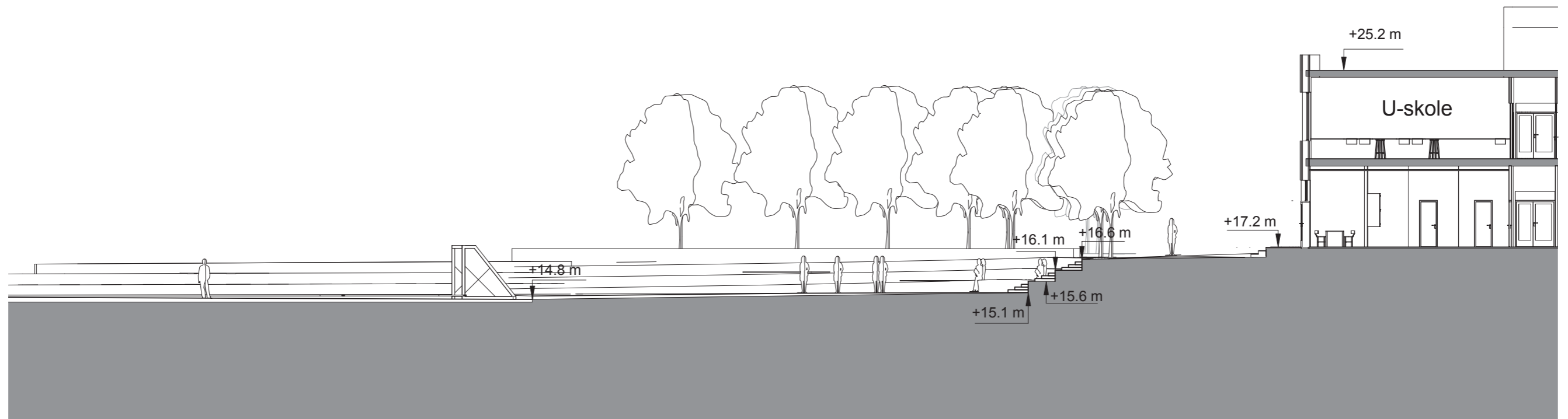
1 Snitt 1 1 : 200
