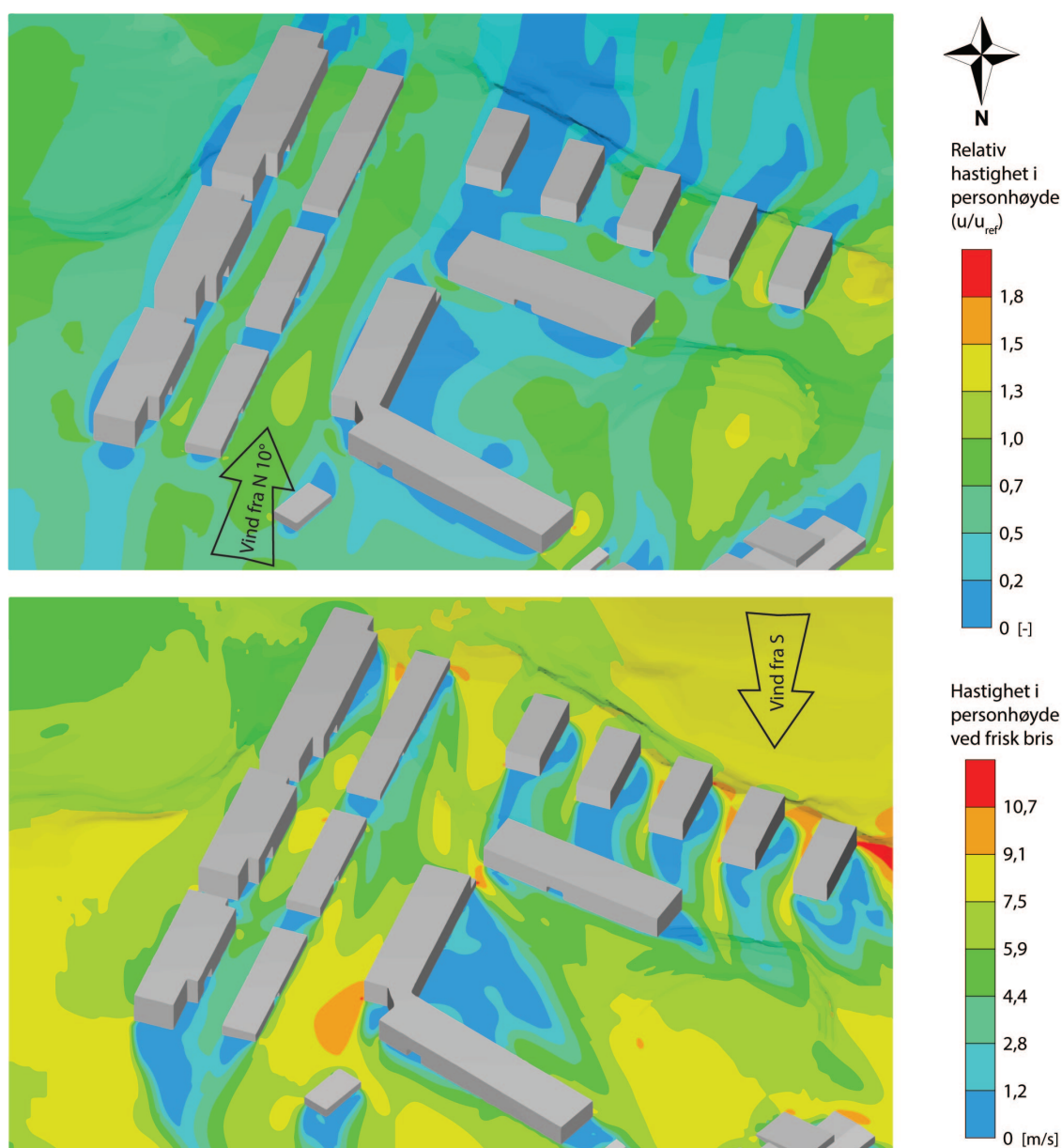
Figur 7. Vindhastigheter i personhøyde rundt aktuelt utbyggingsforslag ved vind fra N (10°) og S (180°).
