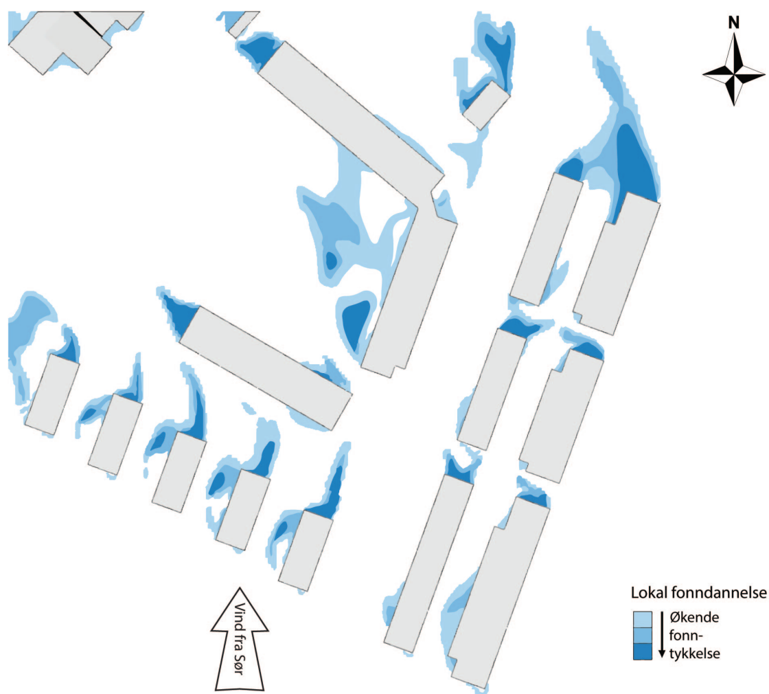
Figur 9. Simulert fonndannelse rundt utbyggingsforslag for B2B, som følge av frisk bris fra S.
