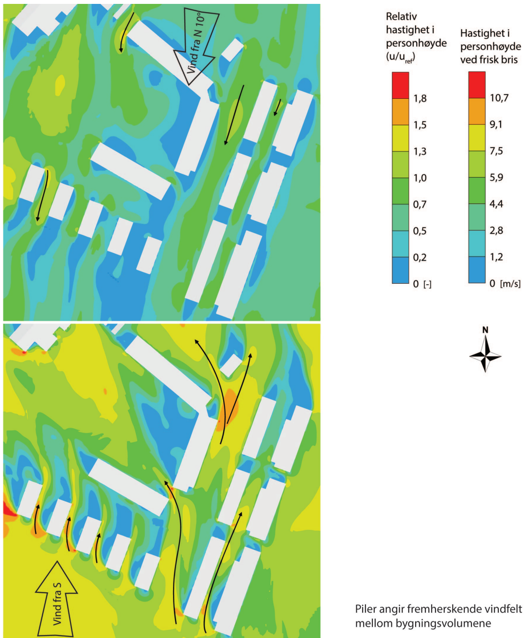
Figur 8. Vindhastigheter i personhøyde rundt aktuelt utbyggingsforslag ved vind fra N (10°) og S (180°) .
